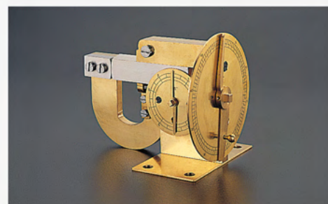
Micrómetro de Watt, 1772
